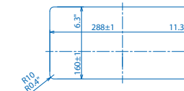
Écran multifonction (encastré) TZT9F Dimensions de découpe
